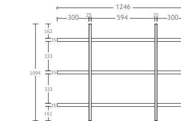
RETROALZATA BOTTIGLIERA "TRALIX" P 270 "TRALIX" BOTTLE COMPARTMENT D 270
