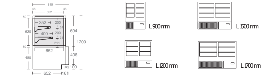
VETRINA REFRIGERATA VENTILATA CON MOTORE INCORPORATO H1350 P827 MM REFRIGERATED VENTILATED DISPLAY CASE WITH HERMETIC UNIT H1200 D827 MM
