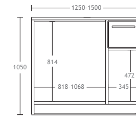
BASE PER MACCHINA CAFFÈ COFFEE MACHINE UNIT
