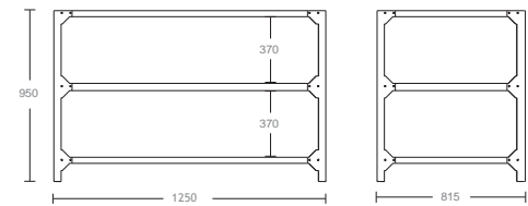
SCAFFALE BASSO A TERRA 1500 P 815 FREE STANDING ISLAND 1500 D 815
