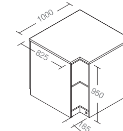
ANGOLO ESTERNO 90° L1000 H950 P1000 MM EXTERNAL CORNER 90° W1000 H950 D1000 MM
