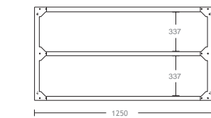
SCAFFALE PENSILE 1500 P 240 WALL SHELF 1500 D 240
