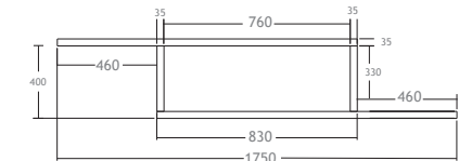
RETROALZATA BOTTIGLIERA ZETA P 236 ZETA BOTTLE COMPARTMENT D 236
