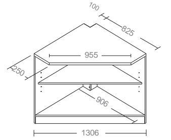
ANGOLO INTERNO 90° L925 H950 P925 MM INTERNAL CORNER 90° W925 H950 D925 MM
