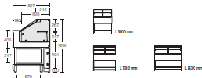
VETRINA CALDO SECCO H1200 P1827 MM HOT DRY DISPLAY CASE H1200 D827 MM
