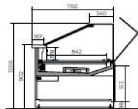
CALDO VENTILATO _ HOT VENTILATED Dim: 1500-2000-2500-3000 mm
