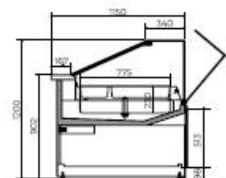
BAGNOMARIA _ DANUBIO Dim: 1500 mm
