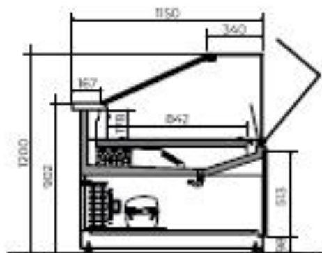
FREDDO VENTILATO _ COLD VENTILATED Dim: 1500-2000-2500-3000 mm
